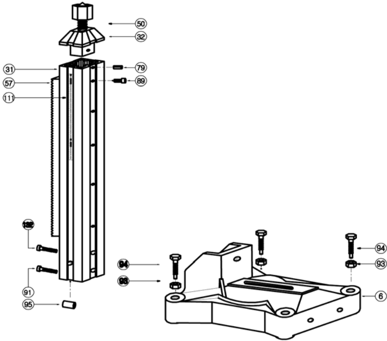
Станина
