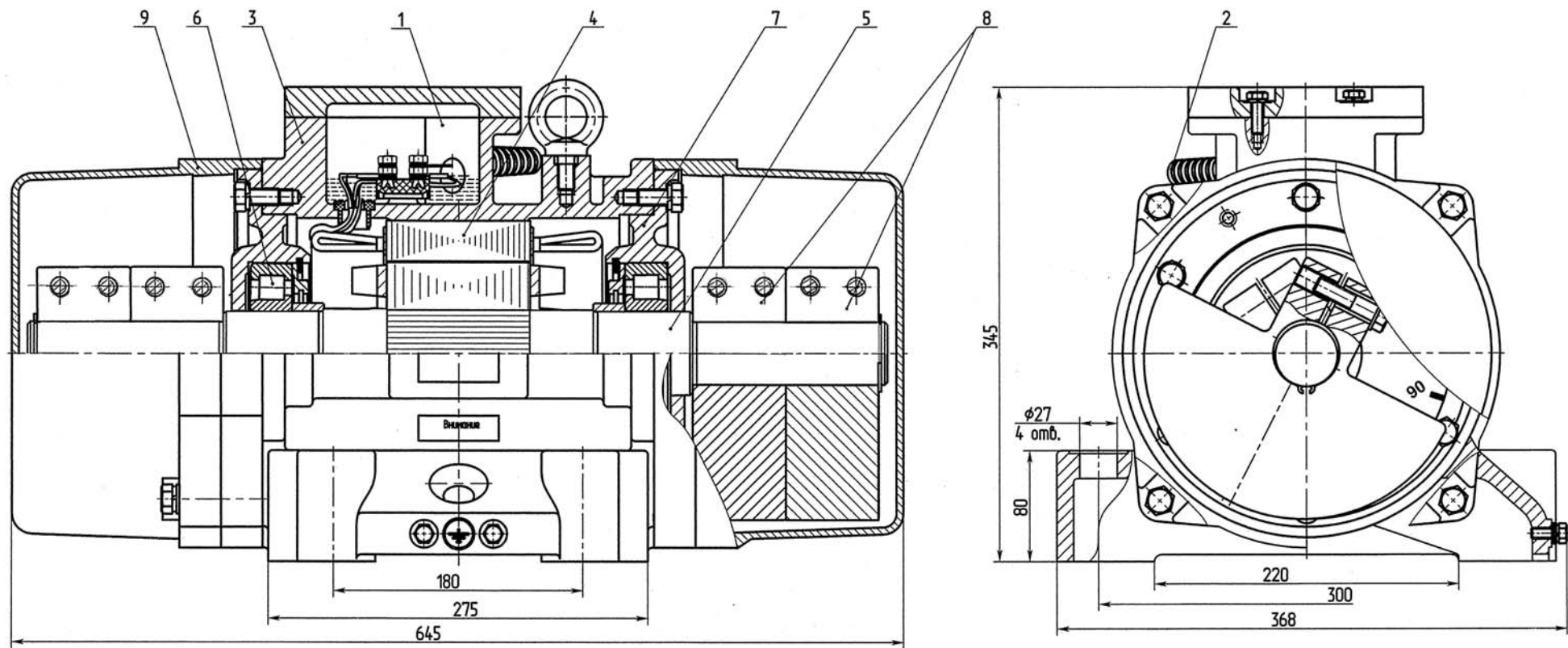
Рисунок 3. Вибратор ИВ-23-16:
