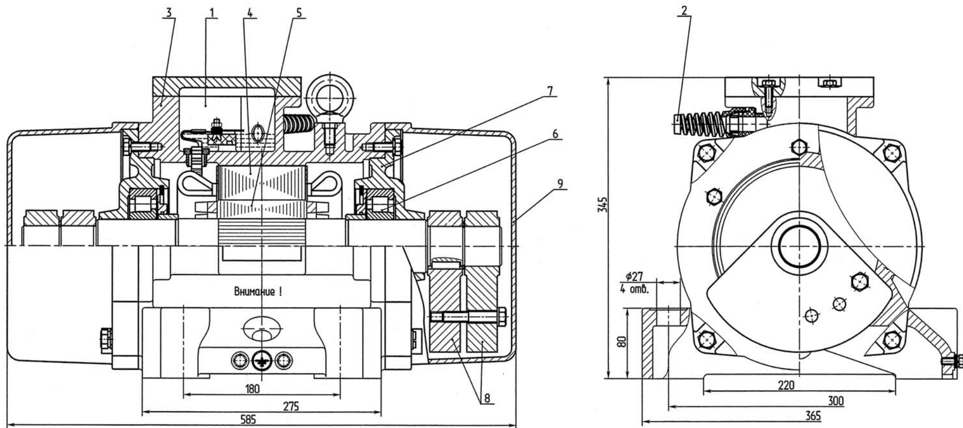
Рисунок 2. Вибратор ИБ-25-25, ИБ-35-25:
