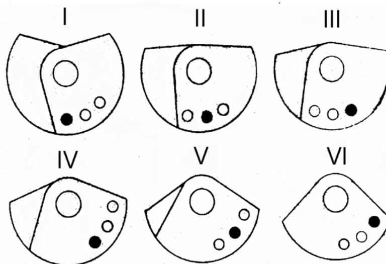
Рисунок 4. Схема регулировки статического момента для ИВ-25-25, ИВ-35-25.
