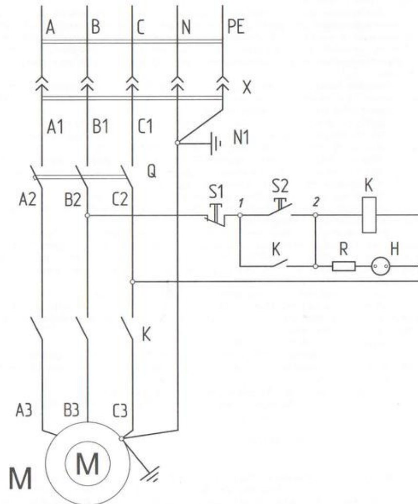
Рисунок 1 - Схема электрическая принципиальная машины СО-307
