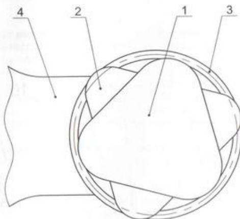
Рисунок 3 – Крепление абразивов
