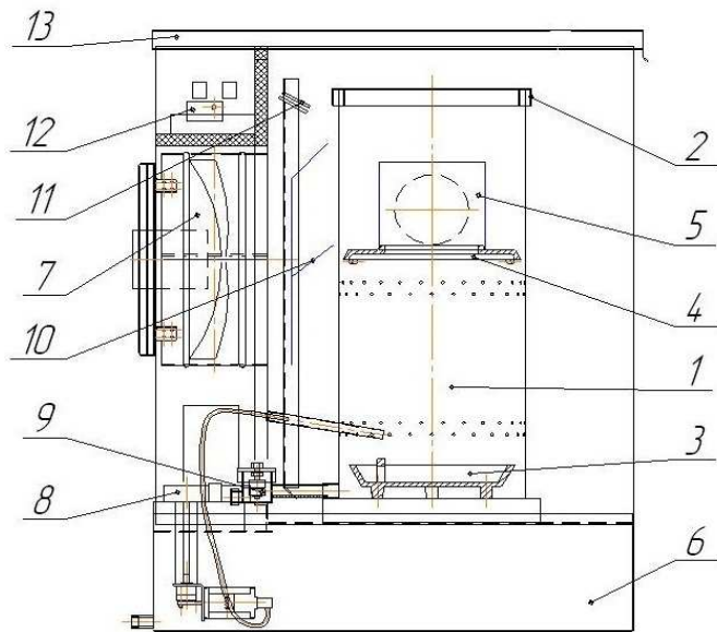
Рис.3 Схема отопителя
